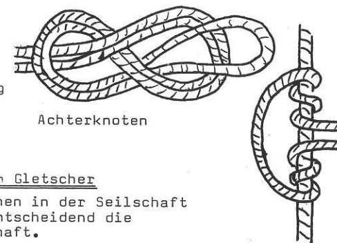
Prusikknoten
